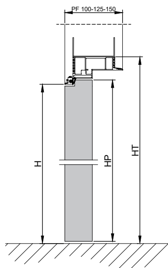
A SPINGERE CON TRAVERSO PUSH WITH UPPER BEAM
